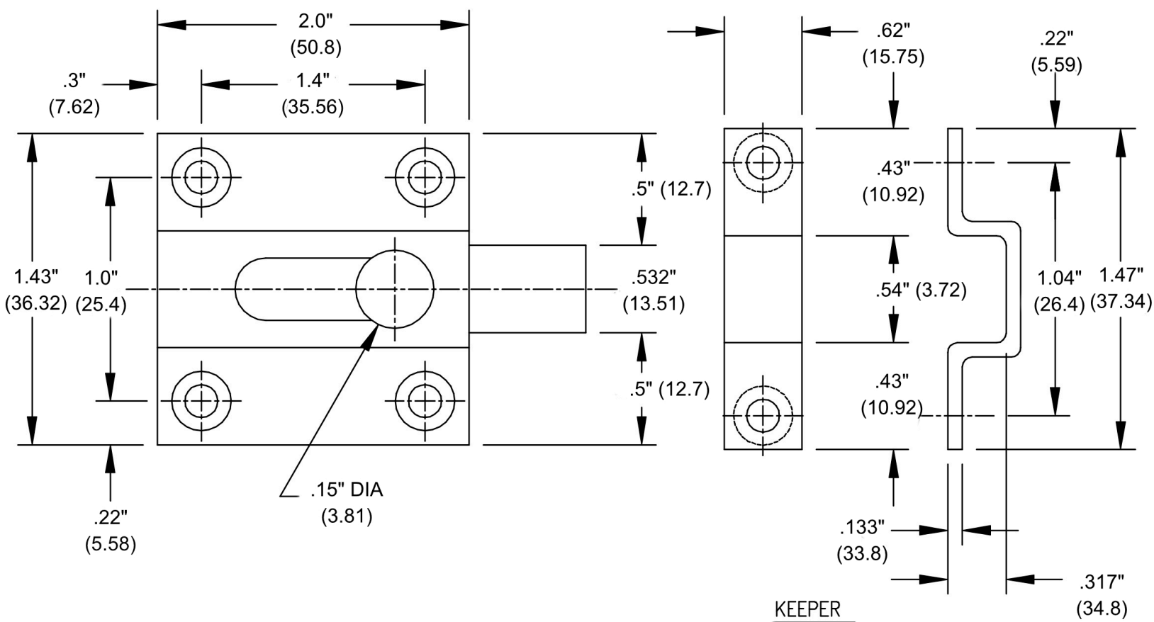
RIM BOLT
